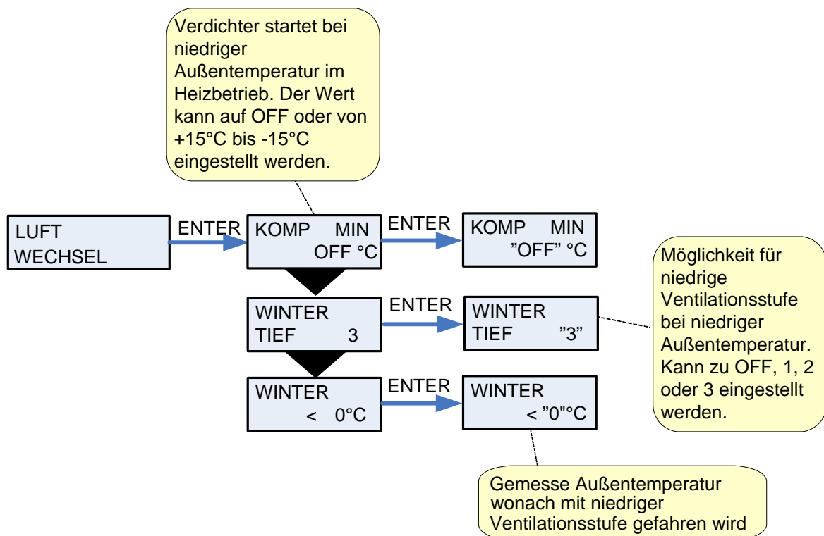
Abbildung 18: Menü „Luftwechsel“
