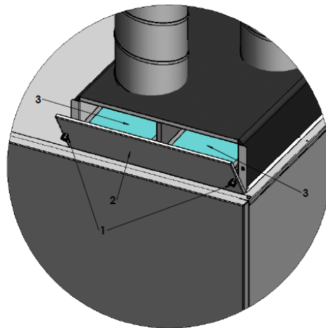
Abbildung 22: Filter wechseln
